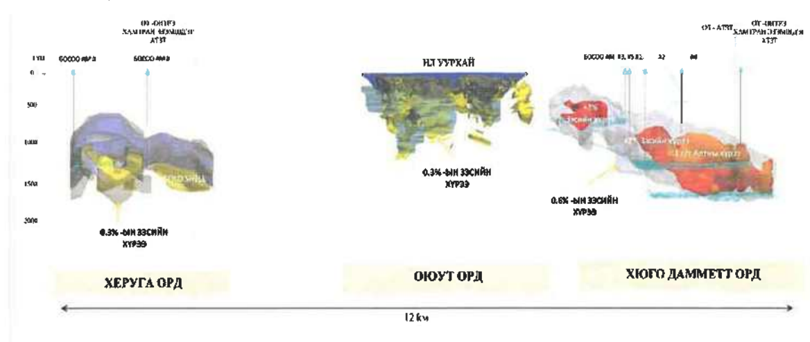
Дүрслэл 1.7. Оюутолгойн бүлэг ордын байршил, зэс болон алтны агуулгуудаар хүрээлсэн тойм зүсэлт, баруун зүгт харсан байдлаар
